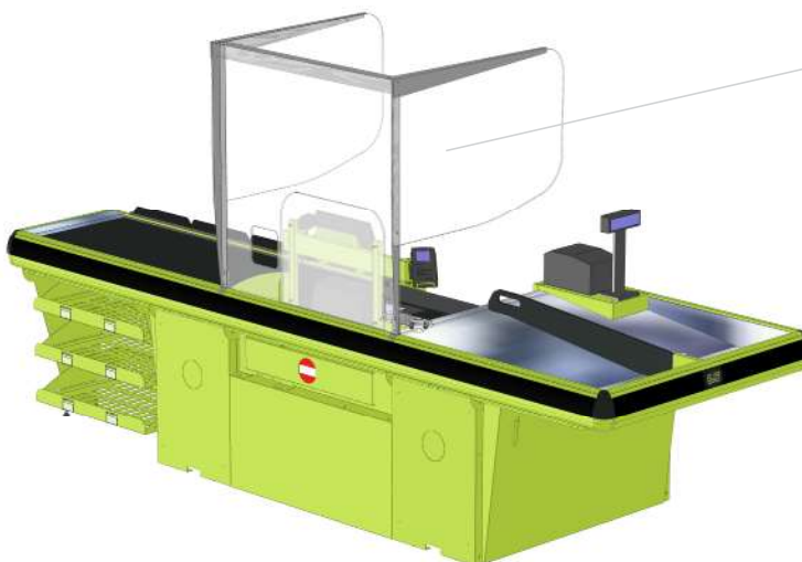
PROTEZIONE CENTRALE con doppio pannello laterale
